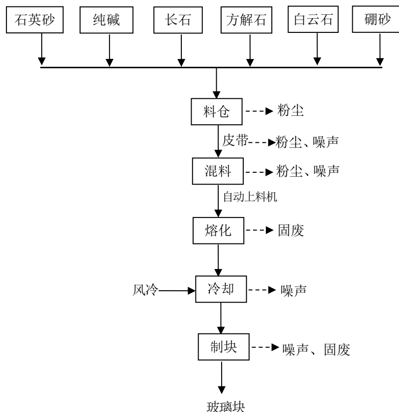
图 2 玻璃料块生产工艺流程图
