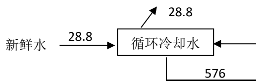
图 1 本项目水平衡图 (单位 m 3 /d)
